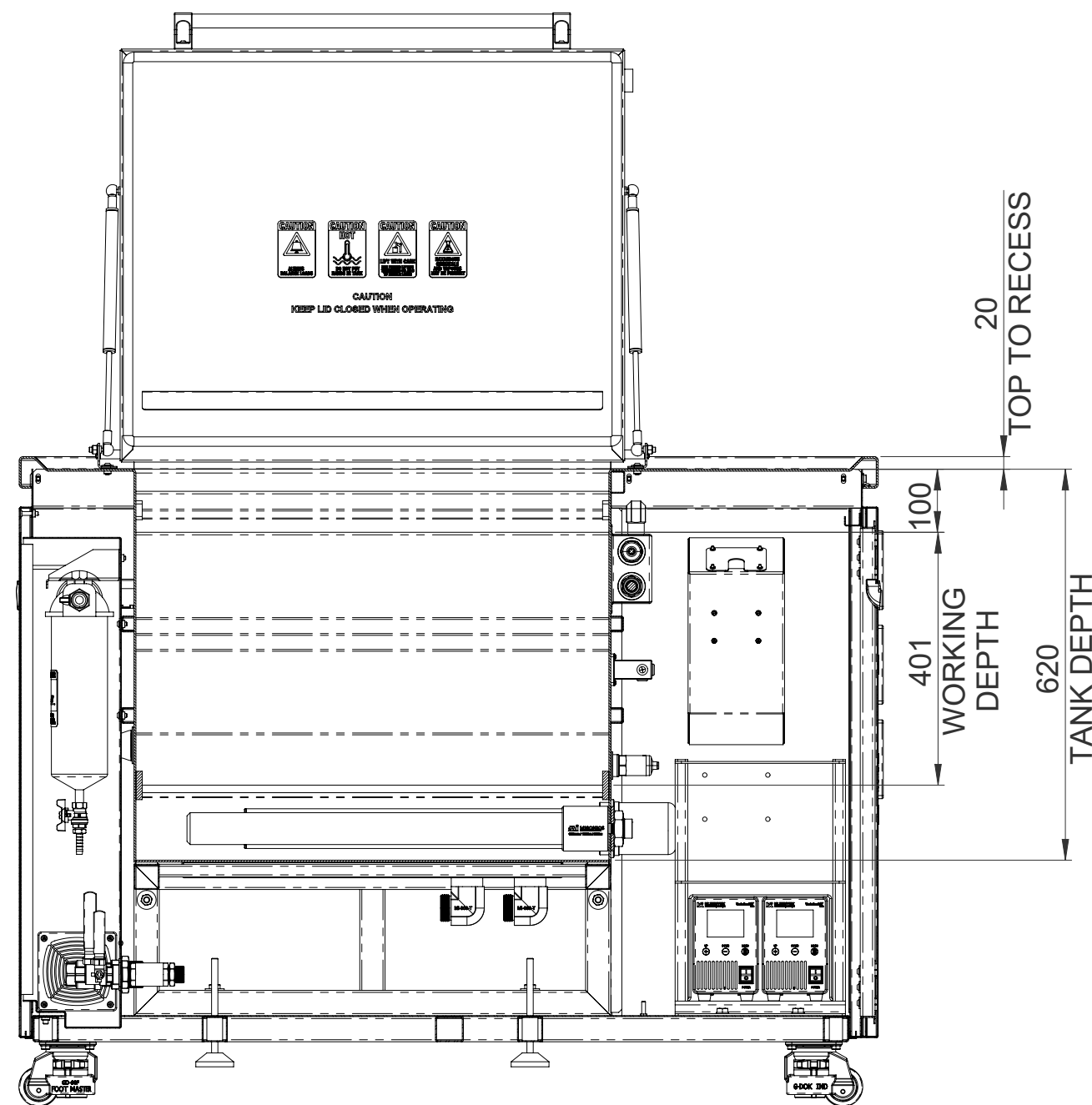
SECTION A-A
